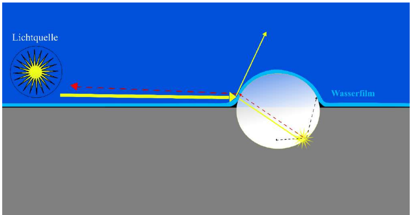
Abb.2 Das Licht wird auf dem Wasserfilm teilweise abgelenkt, so dass weniger Licht in die Perle dringt und retroreflektiert wird.
