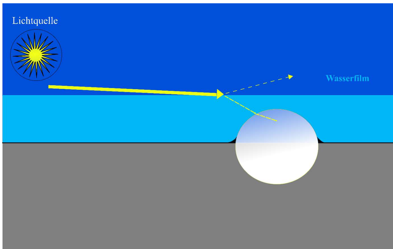
Abb.3 Die Perle wird vom Wasserfilm vollständig überdeckt, so dass das meiste Licht vom Wasserfilm abgelenkt wird. Der noch in die Perle dringende Teil wird dort nicht mehr retroreflektiert, so dass die Markierung nicht mehr gesehen wird.
