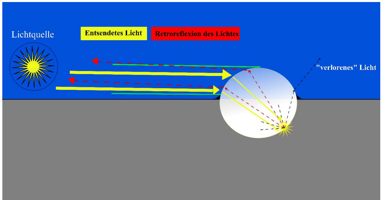
Abb.1 Dargestellt ist der Strahlengang in einer ideal eingebetteten Perle. Ein Teil des Lichtes wird zur Quelle zurückreflektiert.
